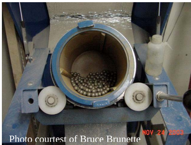
a) Nordic Abrasion Test Drum
