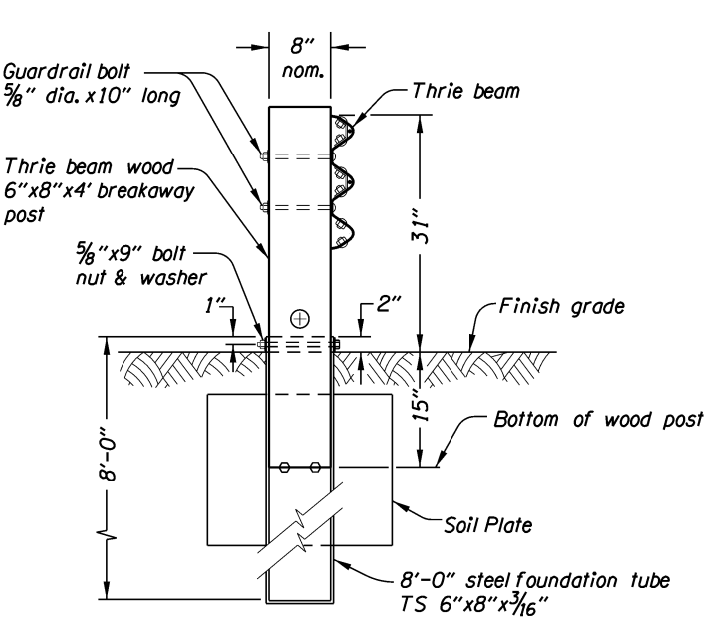
POST 1R & 1L
