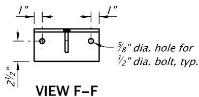
BOTTOM PLATE Scale: 1"=1'-0"
