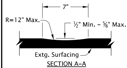
RUMBLE STRIP GROOVE
