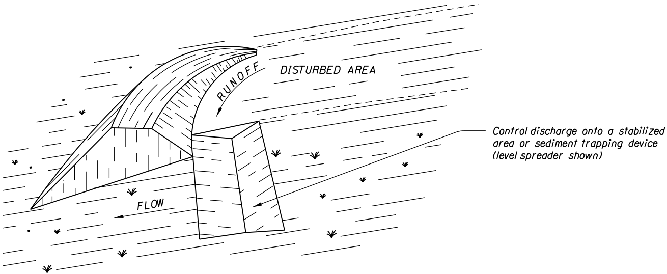
PERIMETER DIKE
