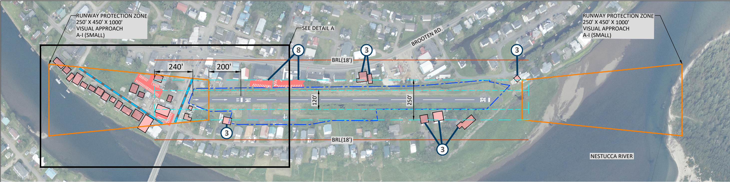
RUNWAY 14-32
