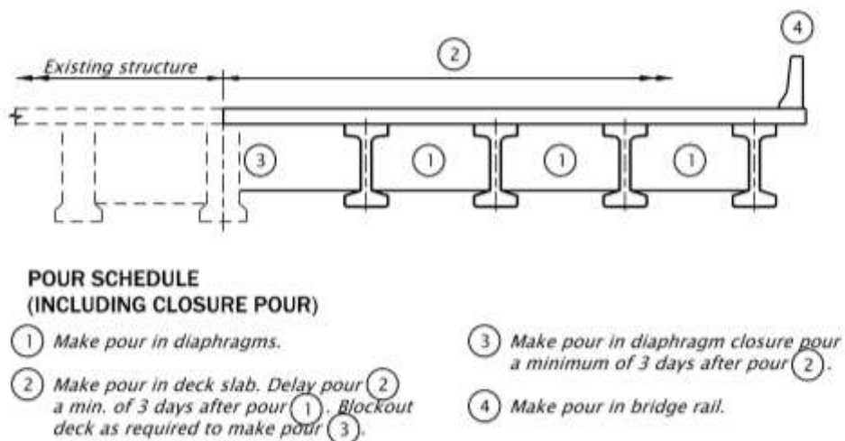
Figure 1.5.6.2.6-2 Delayed Diaphragm Pour Method
