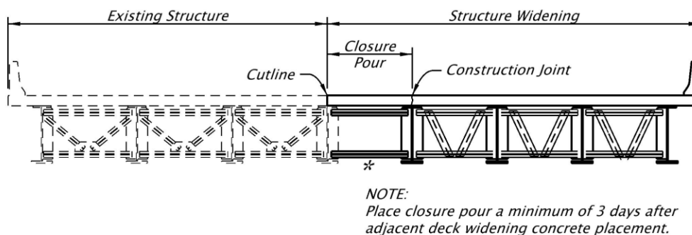
Figure 1.6.2.18-1 Widening Closure Pour Detail
